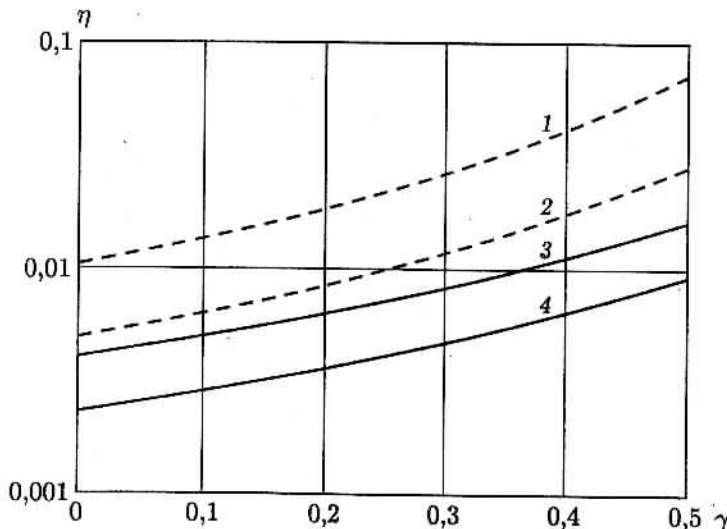
Нормированные рассеяния аппликативной и аддитивной оценок (кривые 1 и 3 рассчитаны при q = 2 , а кривые 2 и 4 — при q = 3 )
