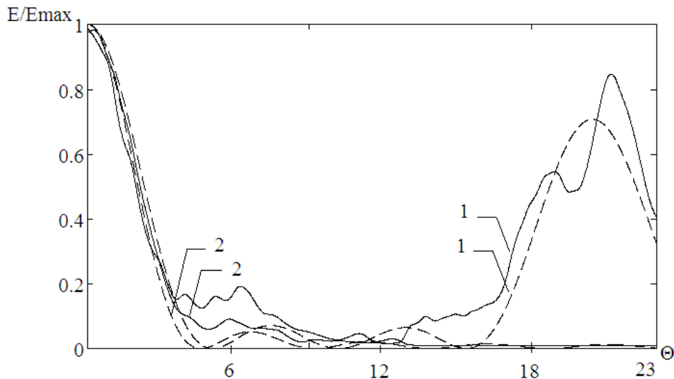
Рис. 3. Нормированные на максимум ДН ДР (переход разреженной решетки в заполненную).
